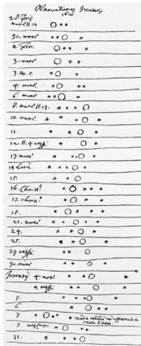
图8 伽利略根据望远镜的观察结果描绘的木星及其卫星
